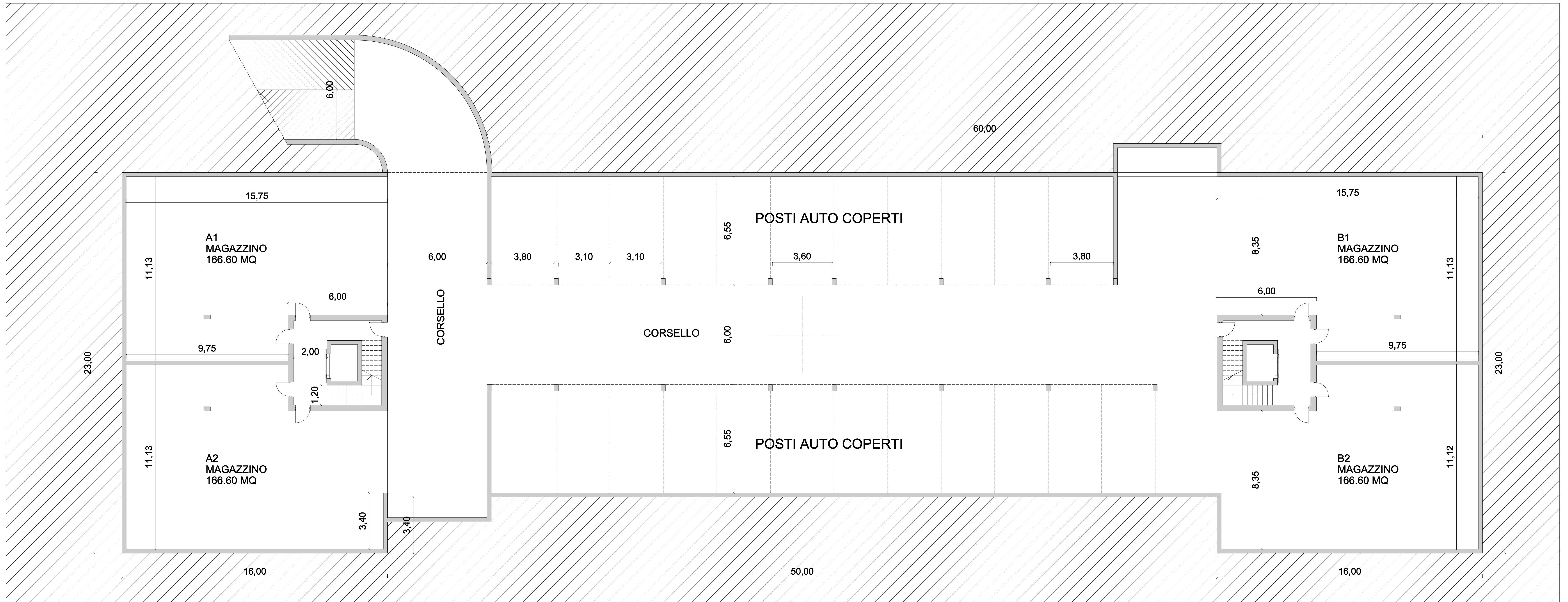
PIANTE PIANO INTERRATO SCALA 1:100 H =2.60
